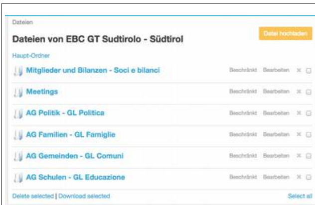
Fig. 12: Dateiordner, Beispiel
