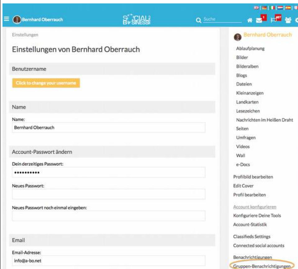
Fig. 6: Gruppen-Benachrichtigungen wählen
